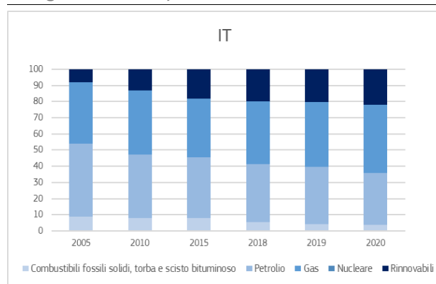
Grafico A5.2 - Energia: quota nel mix energetico (combustibili solidi, petrolio, gas, nucleare, energie rinnovabili)
