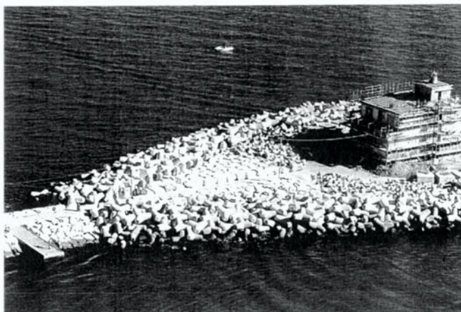
Molo di Malamocco. Lavori per l'adeguamento del faro, al termine degli interventi di ristrutturazione del molo
