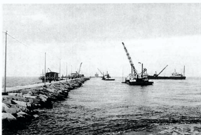
Molo di Malamocco. Un tratto del molo nord all'inizio degli interventi di rinforzo della scogliera
