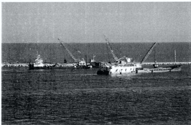
Bocca di Chioggia – Porto rifugio – Scogliera sud
