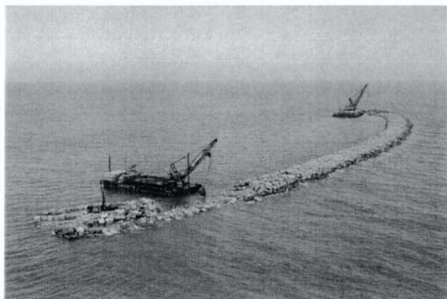
Bocca di Chioggia - Diga foranea. Vista della diga
