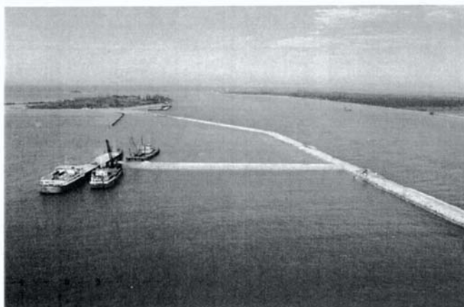
Bocca di Malamocco – Conca di navigazione – camera della conca. Opere provvisionali di protezione dell'area dei lavori
