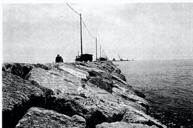
Molo di Malamocco. Un tratto del molo nord al termine degli interventi di rinforzo della scogliera
