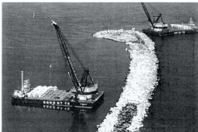
Bocca di Chioggia - Diga foranea. Testata nord, posa degli accropodi
