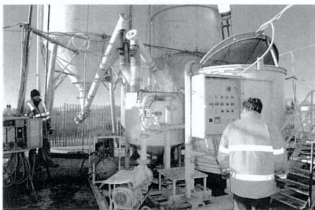
Bocca di Lido - Campo prova dei pali di fondazione. Attrezzature
