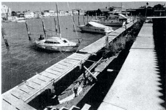
Murano - Canale degli Angeli. La riva prima dei lavori
