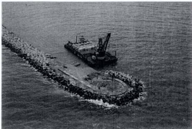
Bocca di Chioggia - Diga Foranea
