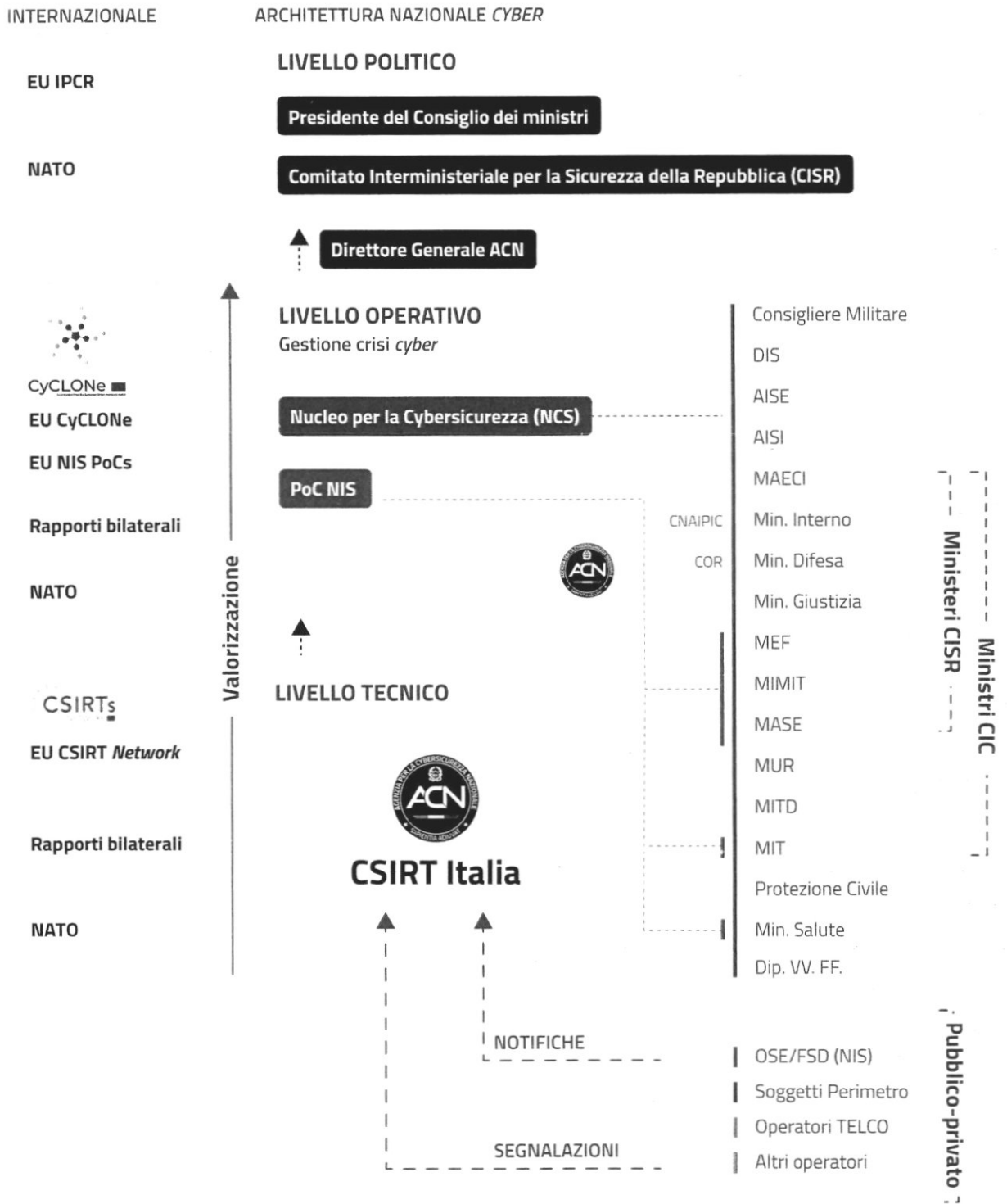
Figura 10: Architettura nazionale cyber e relativo inquadramento nel contesto internazionale e dell'UE
