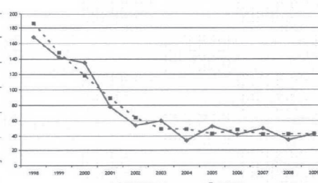
Figura II.25 - DURATA DELLE INTERRUZIONI ACCIDENTALI LUNGHE DEL SERVIZIO ELETTRICO IN BASSA TENSIONE, 1998-2009 (minuti per utente)
