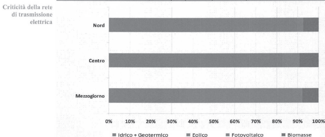
Figura II.24 - POTENZA EFFICIENTE LORDA DELLE FONTI RINNOVABILI PER TIPOLOGIA D'IMPIANTO, 2009 (composizione percentuale)
