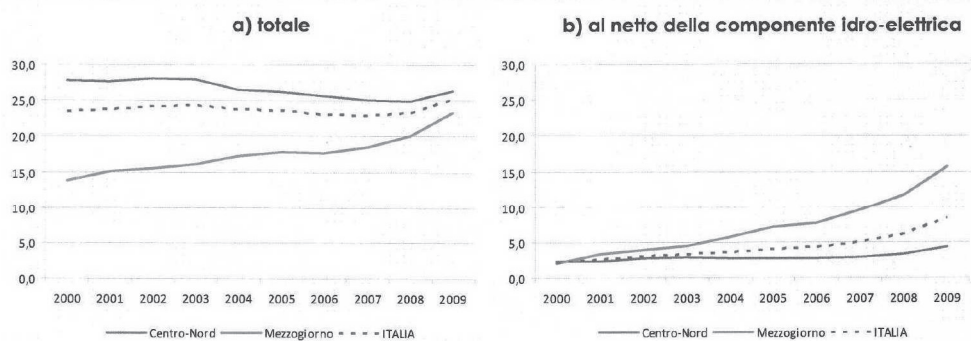
Figura II.23 - POTENZA EFFICIENTE LORDA DELLA GENERAZIONE DA FONTI RINNOVABILI, 2000-2009 (quote percentuali della potenza installata)
