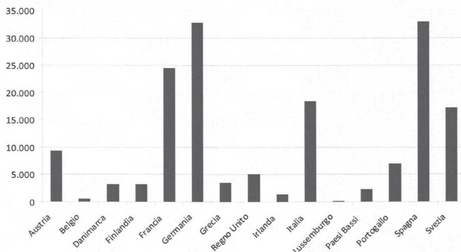
Figura II.22 - UE-15: POTENZA LORDA DEGLI IMPIANTI DI GENERAZIONE CON FONTI RINNOVABILI, 2008 (MW)
