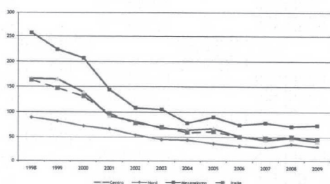
Figura II.25 - DURATA DELLE INTERRUZIONI ACCIDENTALI LUNGHE DEL SERVIZIO ELETTRICO IN BASSA TENSIONE, 1998-2009 (minuti per utente)
