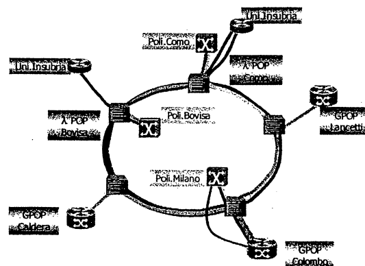
Anello Ottico Milano-Como nella Rete regionale dell'Insubria
