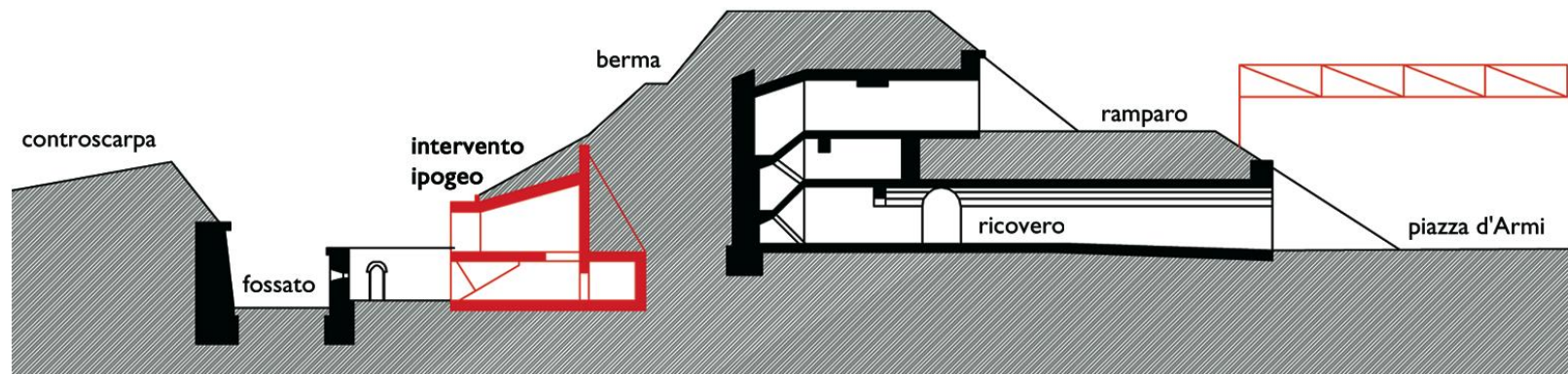
SEZIONE DELLO STATO DI FATTO E DI PROGETTO CON AMPLIAMENTO IPOGEO DEL FORTE
