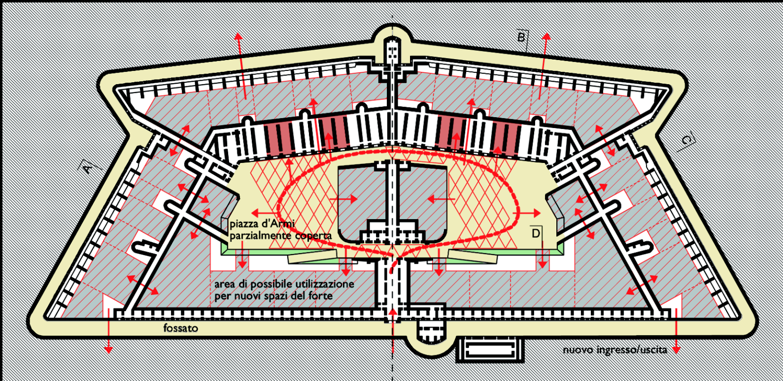
SCHEMA DI REVISIONE DISTRIBUTIVA E AMPLIAMENTO DEL FORTE
